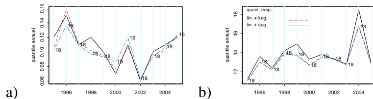
Figure 6. Estimation du quantile 90, à la station 26000 sur la Loire : SEQ-eau (trait plein), et interpolation de la fonction de quantile empirique avec pondération par krigeage ou par segment d'influence. Le nombre de mesures annuelles est reporté. a) nitrites et b) nitrates.
