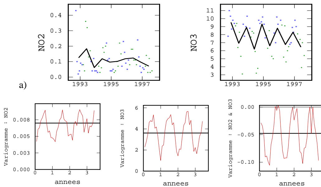
Figure 1. Concentrations en nitrites \text{NO}_2 et en nitrates \text{NO}_3 à la station 6027000 sur le Doubs. a) * mesures de septembre à février, + mesures de mars à août. La courbe correspond aux moyennes semestrielles. b) variogrammes temporels simples et croisés. Le variogramme croisé, négatif dans ce cas, indique l'anticorrélation temporelle des concentrations.
